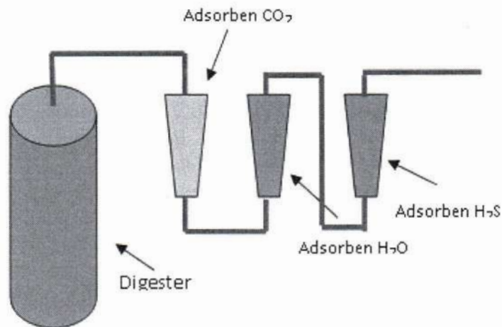
Gambar 1. Digester terintegrasi dengan SAKTI
